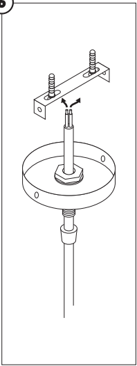
Ledning installeres i eksisterende loftudtag. Wiring installed in existing ceiling sockets.
